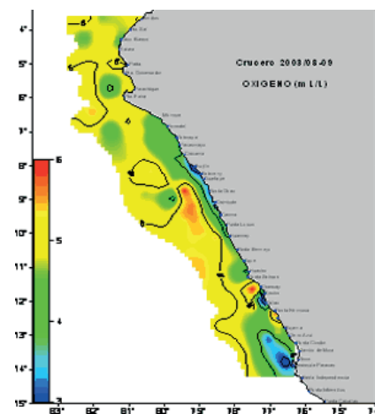
Fig.N°10: Distribución Oxígeno Disuelto (Imarpe)
