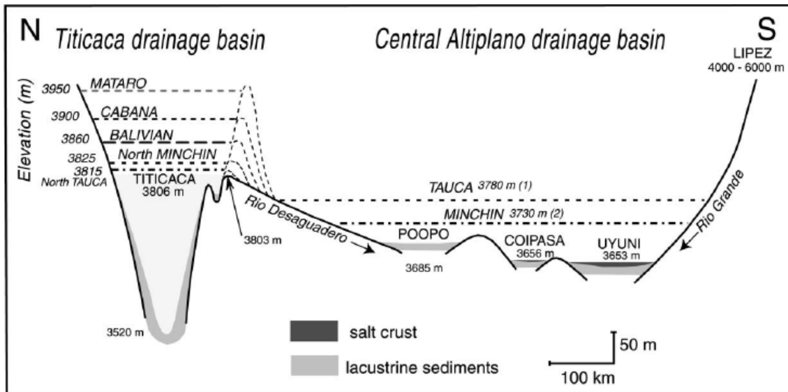
Figura 2. Sección esquemática NS del Altiplano mostrando una reconstrucción de los niveles de los paleolagos en las cuencas del Norte y del Centro (tomado de Fornari et al. , 2001).
